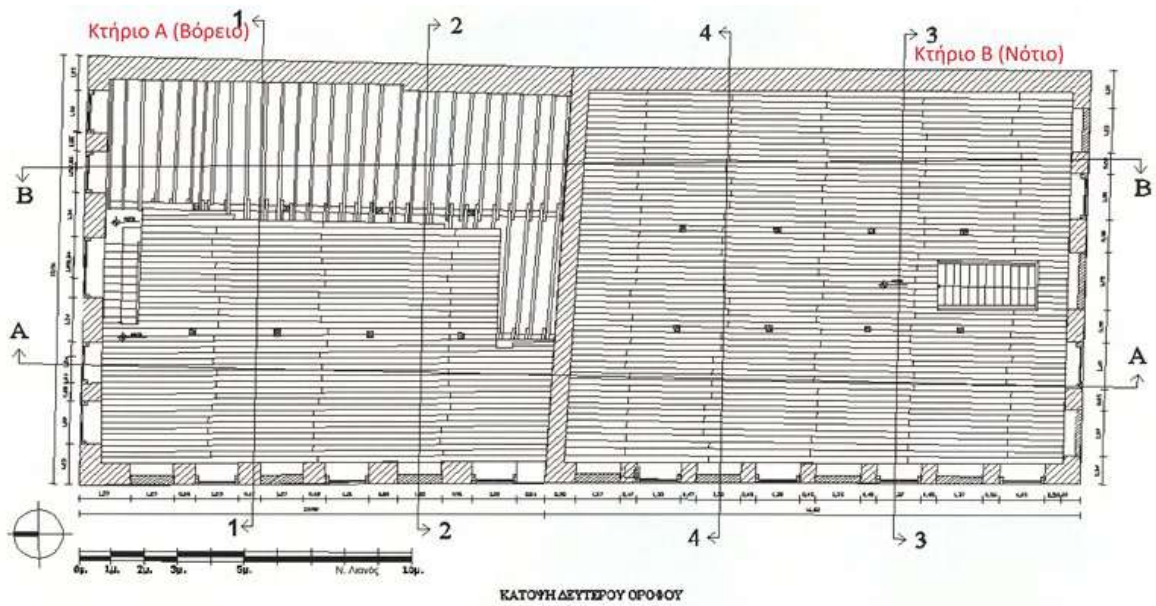
Εικόνα 54 Κάτοψη των δύο κτιρίων στο επίπεδο του ορόφου
