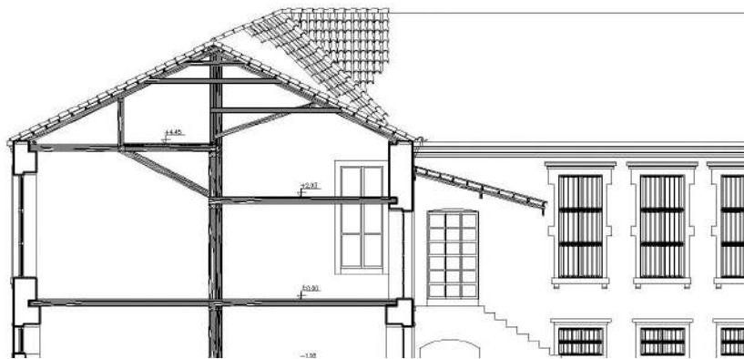
Εικόνα. 14 Σχέδιο τομής του κτιρίου καπναποθήκης(πηγή: Αρχείο ΥΝΜΤΕΑΜΘ)
