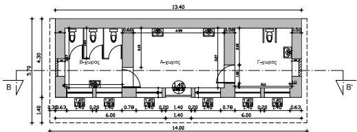
ΚΑΤΟΨΗ ΙΣΟΓΕΙΟΥ
