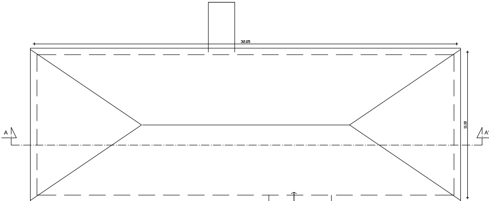
ΚΑΤΟΨΗ ΣΤΕΓΗΣ
