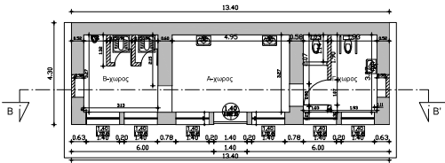
ΚΑΤΟΨΗ ΙΣΟΓΕΙΟΥ / αποτύπωση
